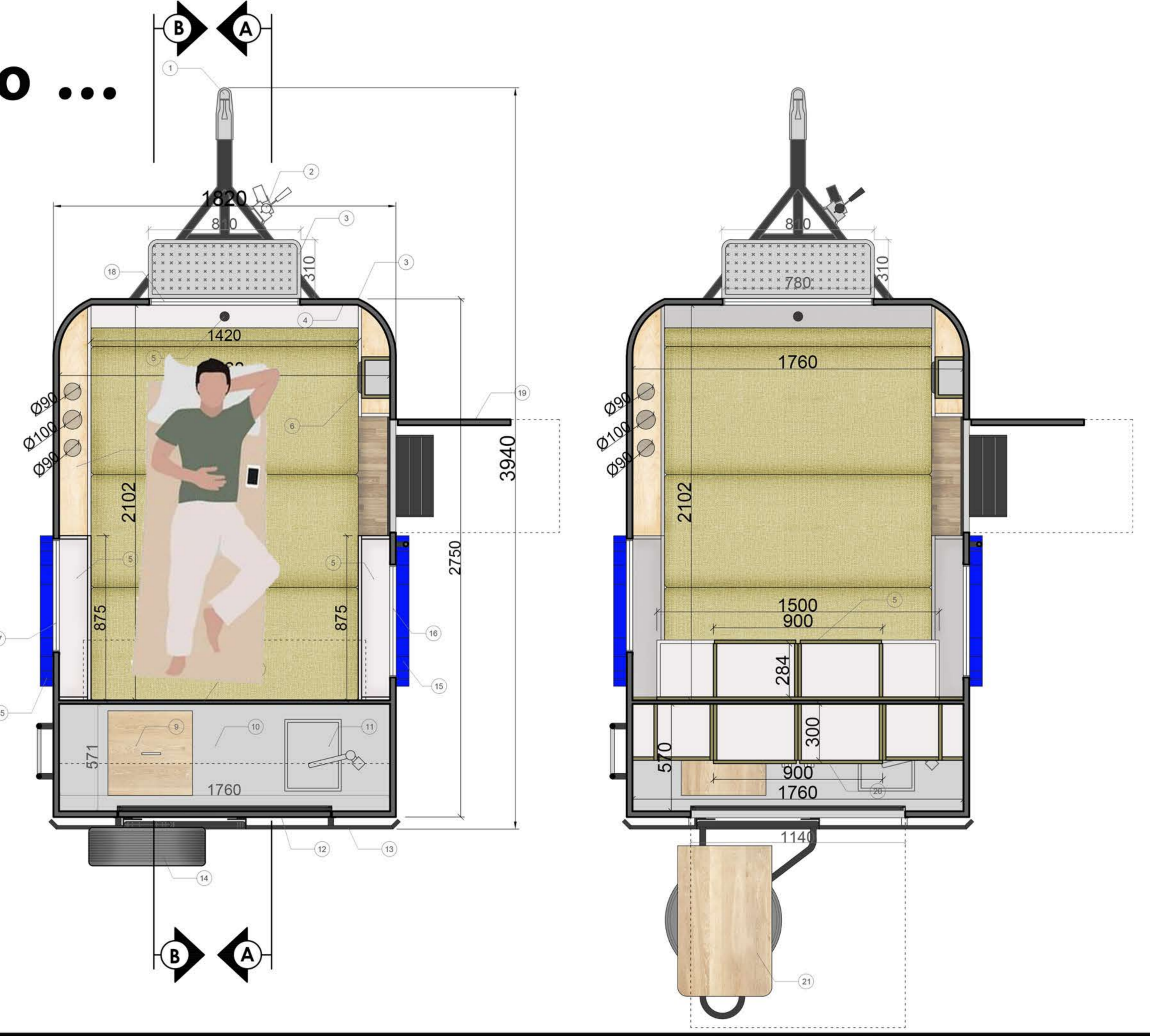
Planta - Nivel 1,6 m
